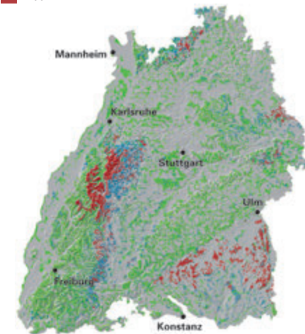
Sturmschadensanfälligkeit für Wälder in Baden-Württemberg auf der Basis der Winterstürme Wiebke und Lothar.
